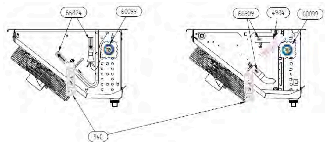
Ansicht Anschlussseite für HFKW und CO 2 (links) bzw. für Glykol (rechts)
