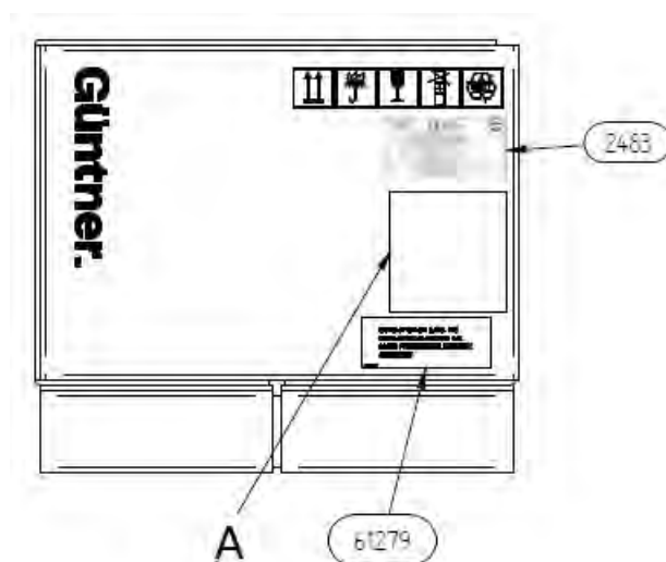
Verpackung Seitenansicht
