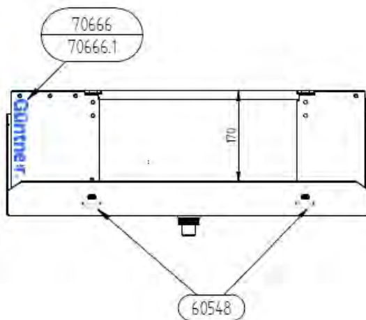
Ansicht Rückseite GASC 020.1
